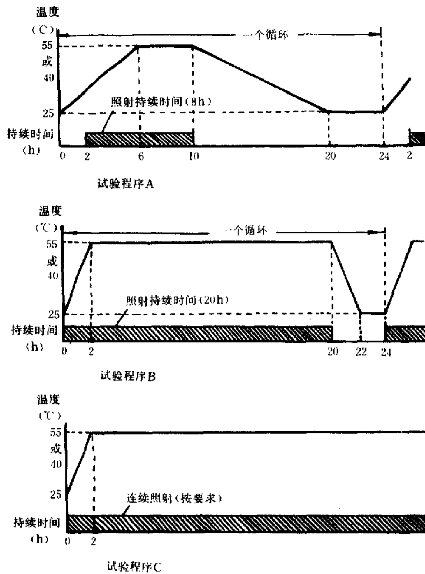
图1 温度-辐照-时间关系图
